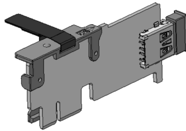
图 39: 内部 USB 3.0 卡, 大小为 40 x 16 x 8 毫米 (L x W x H)
