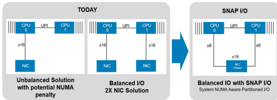
图 15: 将不平衡的单 NIC 解决方案和平衡的双 NIC 解决方案与 SNAP I/O 单 NIC 解决方案进行比较。
