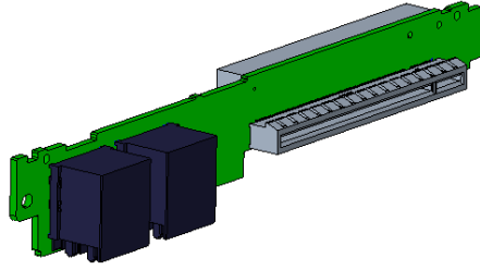
图 19: R1 Paddle (将 PCIe 通道路由至正面背板以用于额外的 NVMe)
