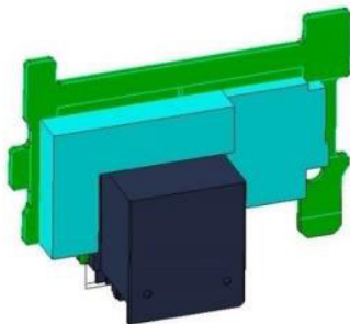
图 24: R3 Paddle (将 PCIe 通道路由至正面背板以用于额外的 NVMe)
