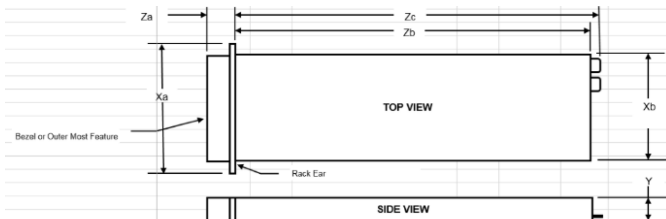
图 36: 机箱尺寸
