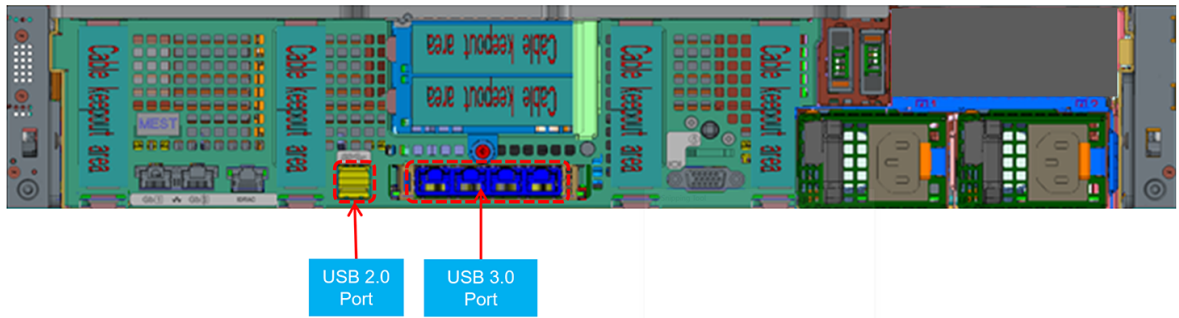
图 20: 背面 USB 3.0 端口（底部）和 USB 2.0 端口（顶部）
