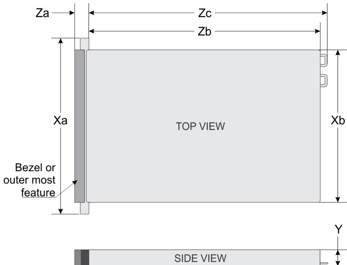
图 18: PowerEdge R550 机箱尺寸
