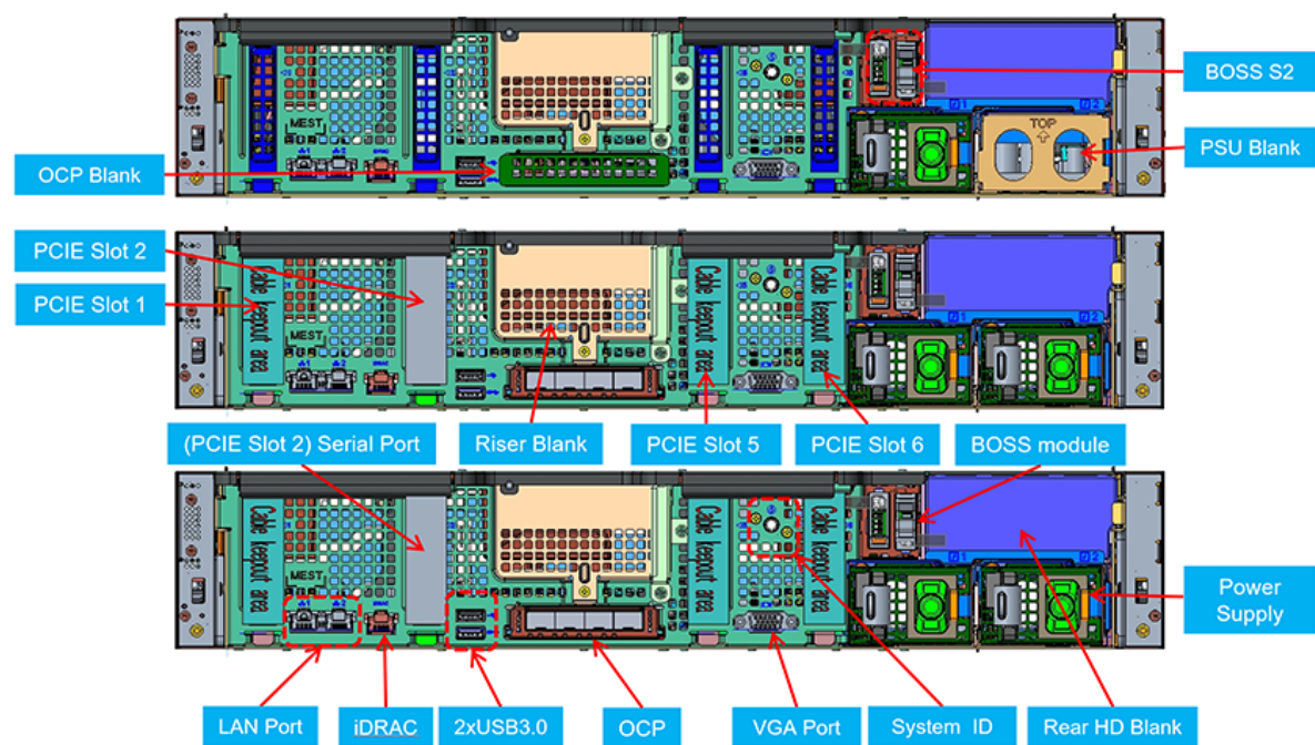
图 4: 系统的后视图
