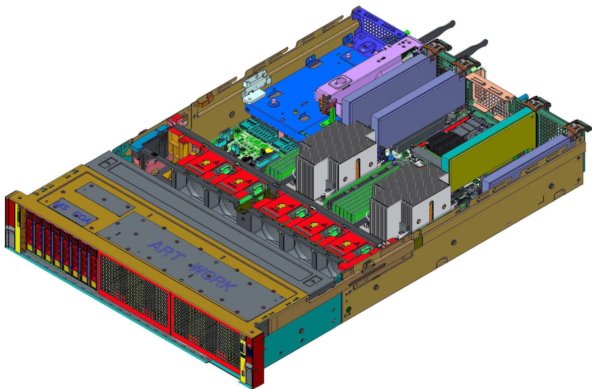
图 5: 系统内部 - 8 x 2.5 英寸
