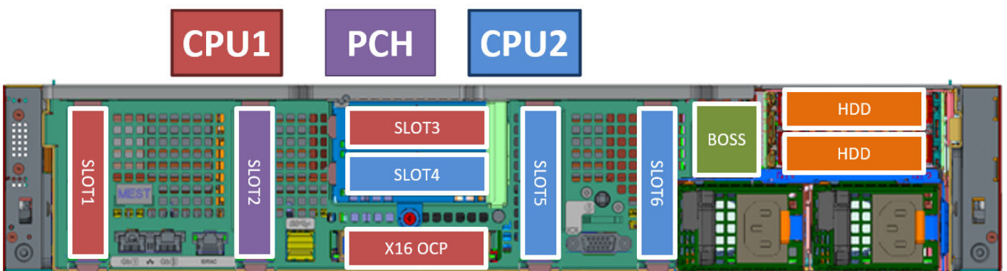
그림 7 . 시스템의 후면
