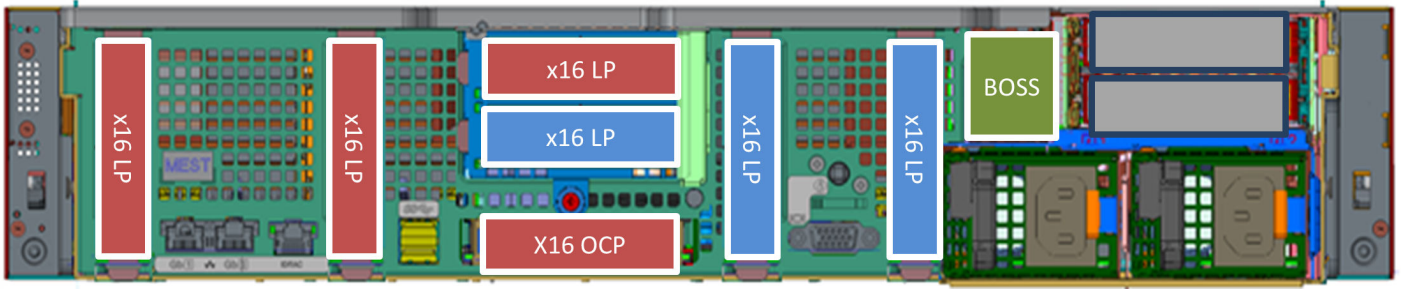
그림 8 . 라이저 슬롯 번호가 있는 시스템의 후면 모습
