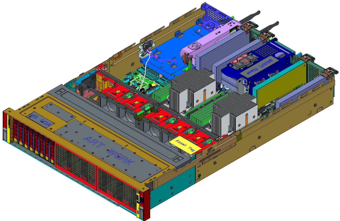
그림 13 . 8개의 2.5" 시스템 내부
