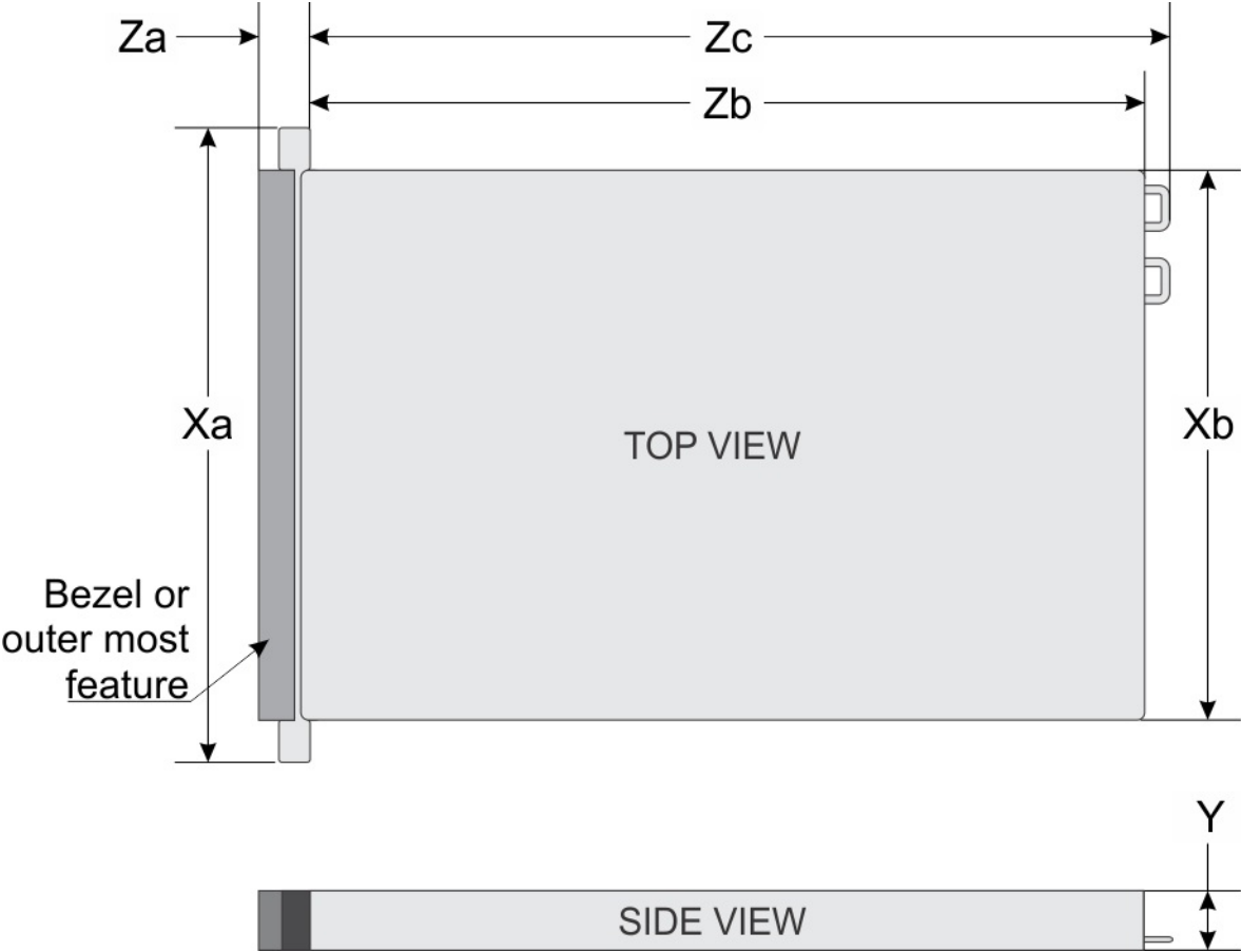
Figure 18. Dimensions du boîtier PowerEdge R450
