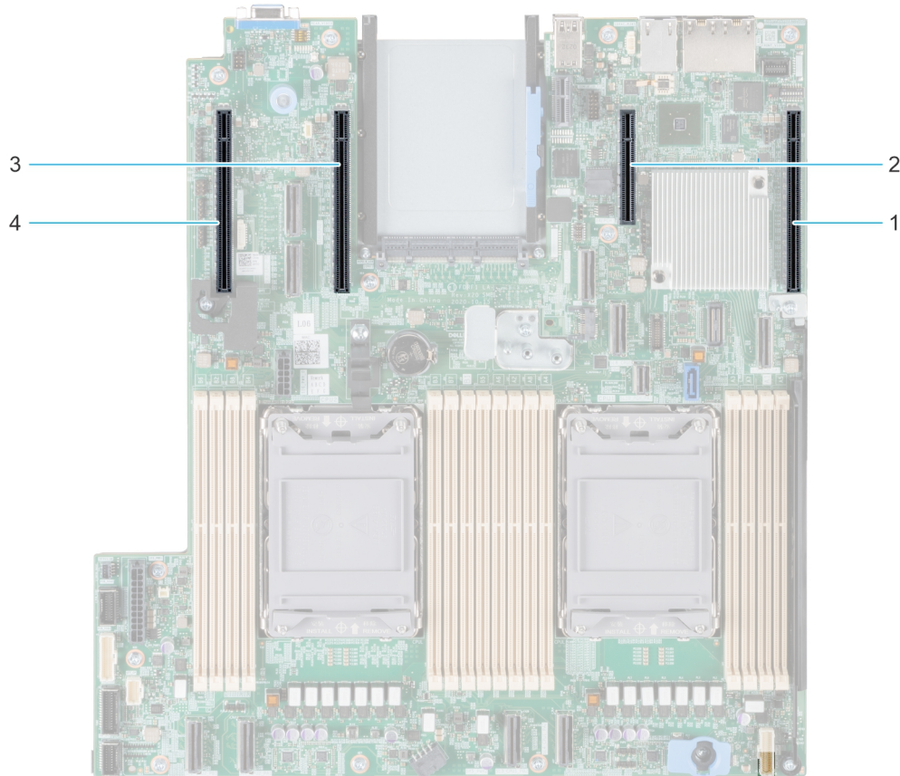
Figure 8. Connecteurs des logements de carte d'extension
